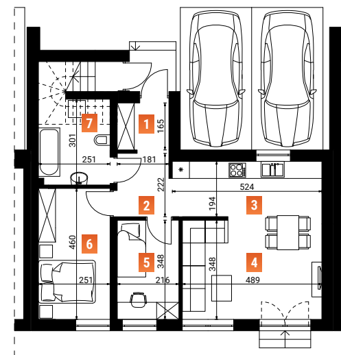
Rzut lokalu
